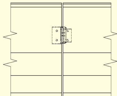
Verbindungselement für zwei Brücken
